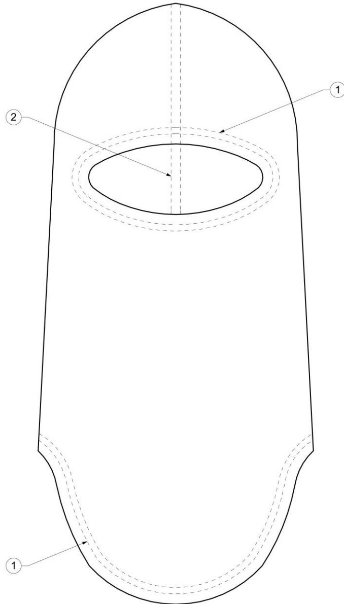
Рисунок Б5.1 — Позначення строчок виробу
