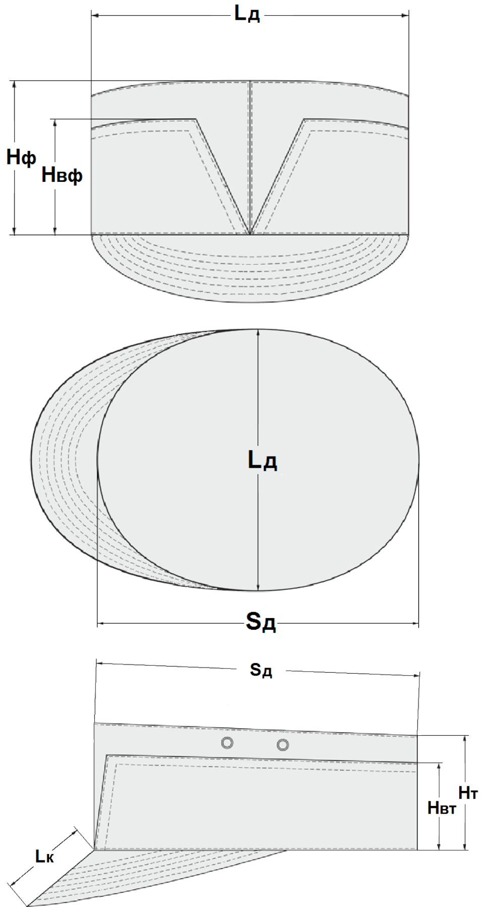
Рисунок 2 – Виміри виробу
