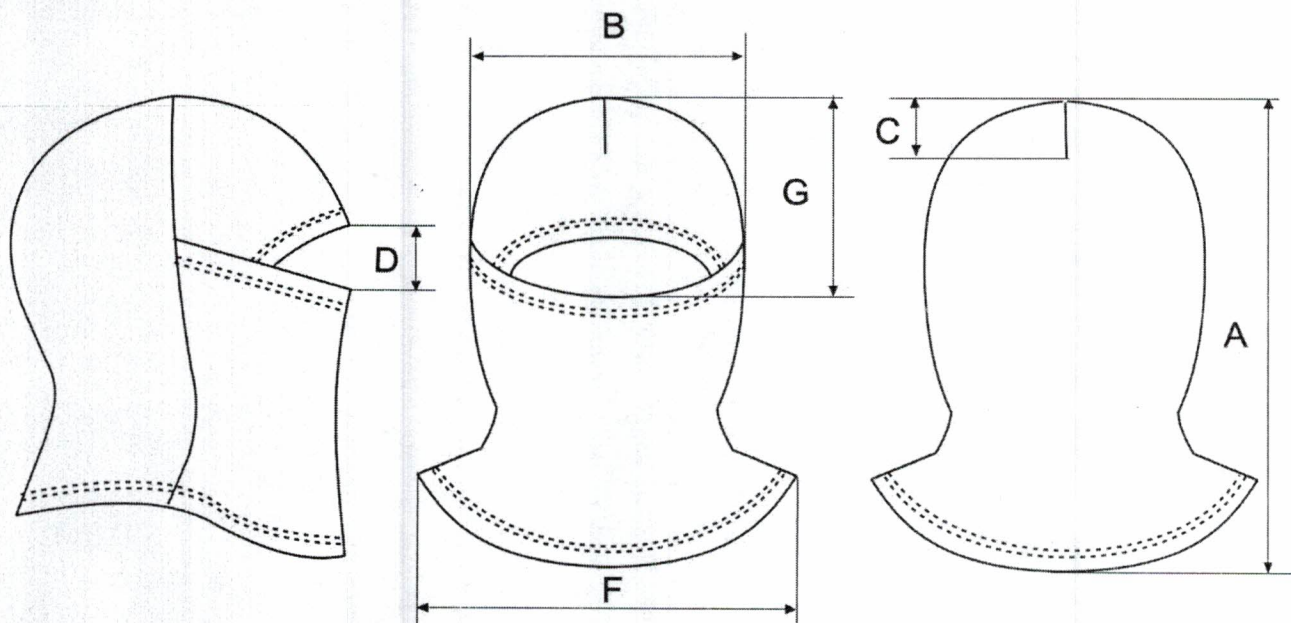
Рисунок Д2.1– Місця лінійних вимірів предмета
