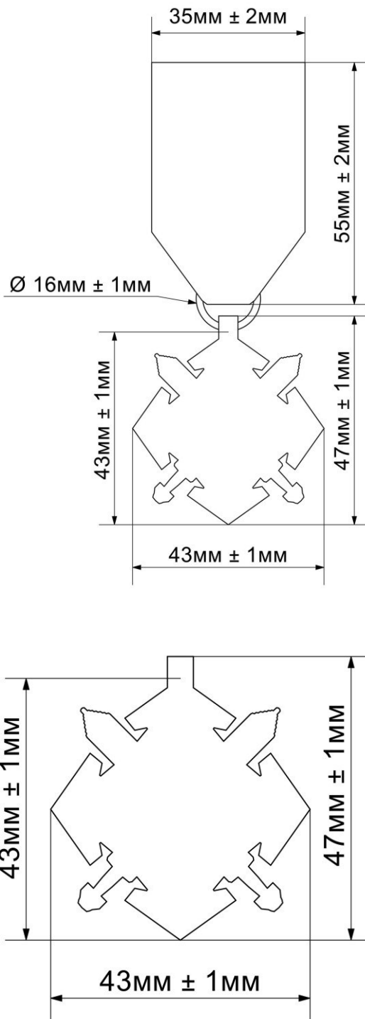
Рисунок Д2.1 – Лінійні розміри предмета
