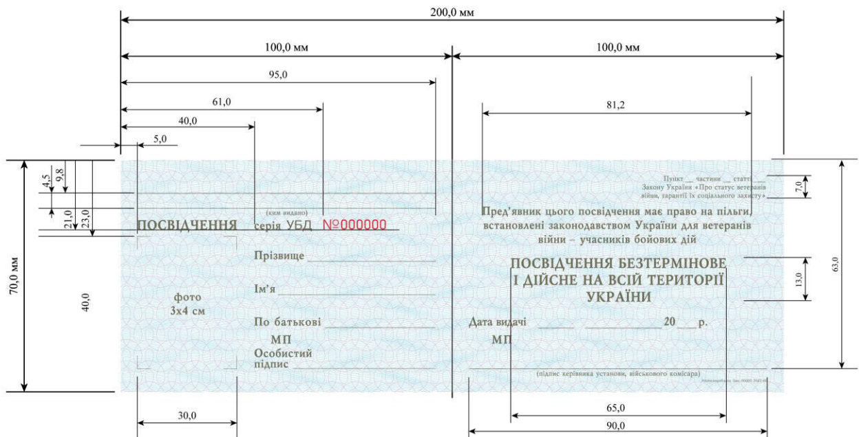
Рисунок Д1.2 – Зовнішній вигляд та лінійні розміри внутрішньої частини предмета у розгорнутому вигляді
