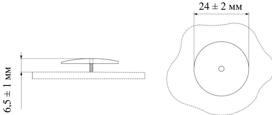
Рисунок Д2.1 – Розміри гвинта із закруткою
