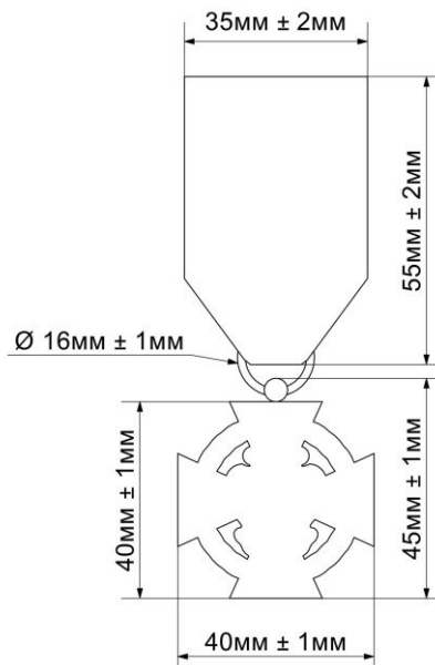
Рисунок Д1.2 – Лінійні розміри предмета
