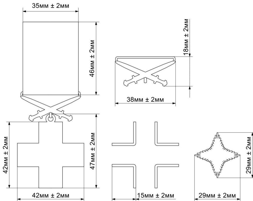
Рисунок Д1.3 – Лінійні розміри предмета
