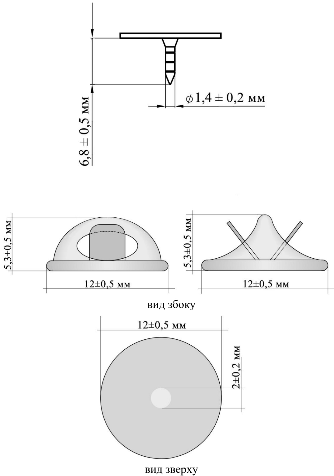
Рисунок Д2.1 – Розміри кріплення
