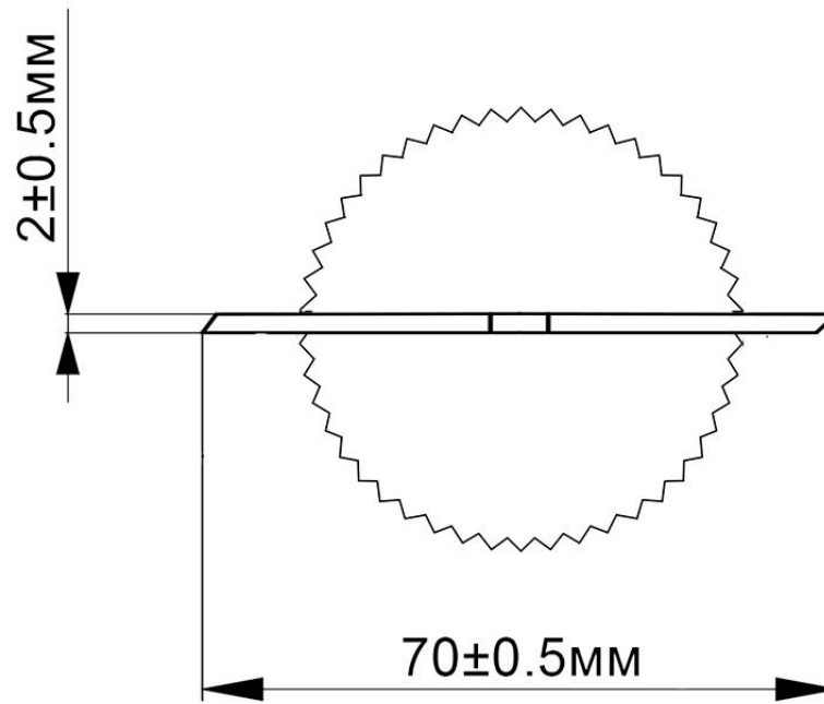
Рисунок Д2.1 – Розміри кріплення
