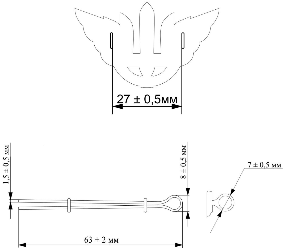
Рисунок Д2.1 – Розміри кріплення
