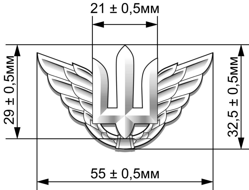
Рисунок Д1.1 – Розміри предмета
