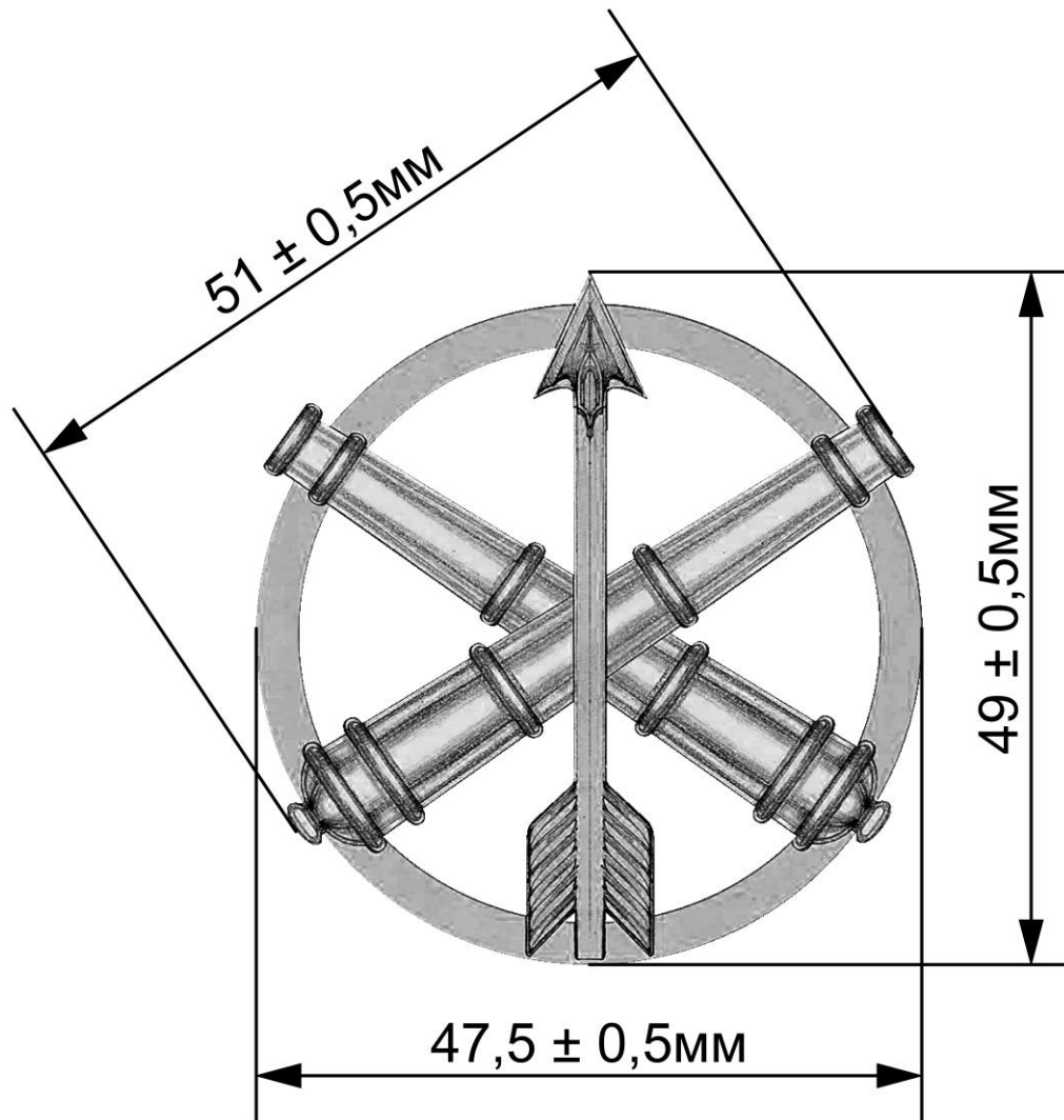
Рисунок Д1.1 – Розміри предмета
