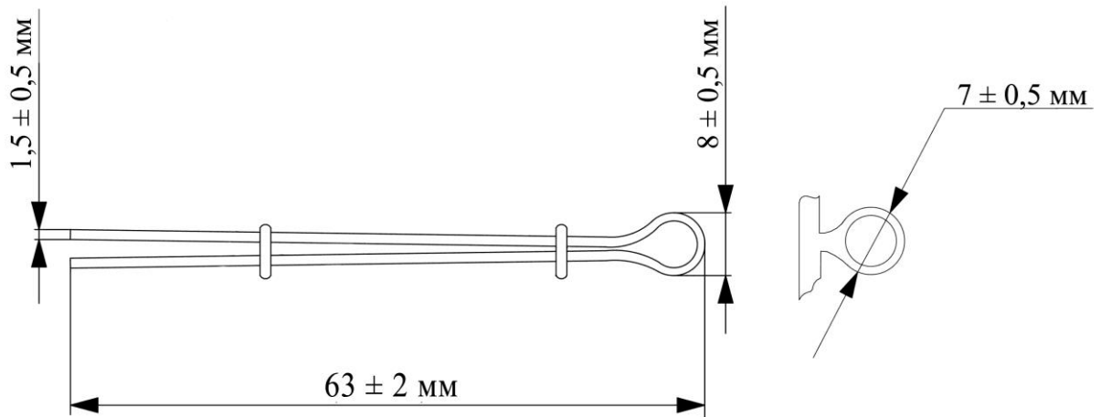
Рисунок Д2.1 – Розміри шпильки
