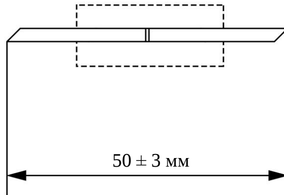
Рисунок Д2.2 – Розміри клямера
