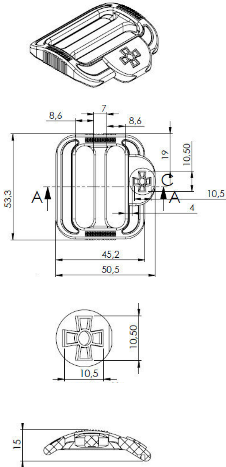
Рисунок Д1.3 – Загальні та лінійні виміри пряжки з логотипом (допустимі відхилення за лінійними відхиленнями пряжки \pm 5\% )
