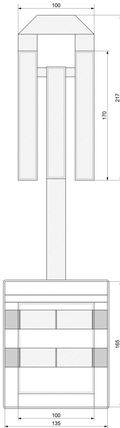
Рисунок Д1.1 – Орієнтовний зовнішній вигляд фронтальної частини предмета
