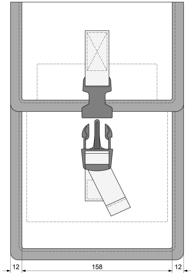
Рисунок Д1.1 – Орієнтовний зовнішній вигляд предмета
