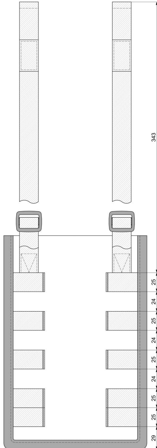
Рисунок Д1.3 – Конструкция зворотного боку предмета
