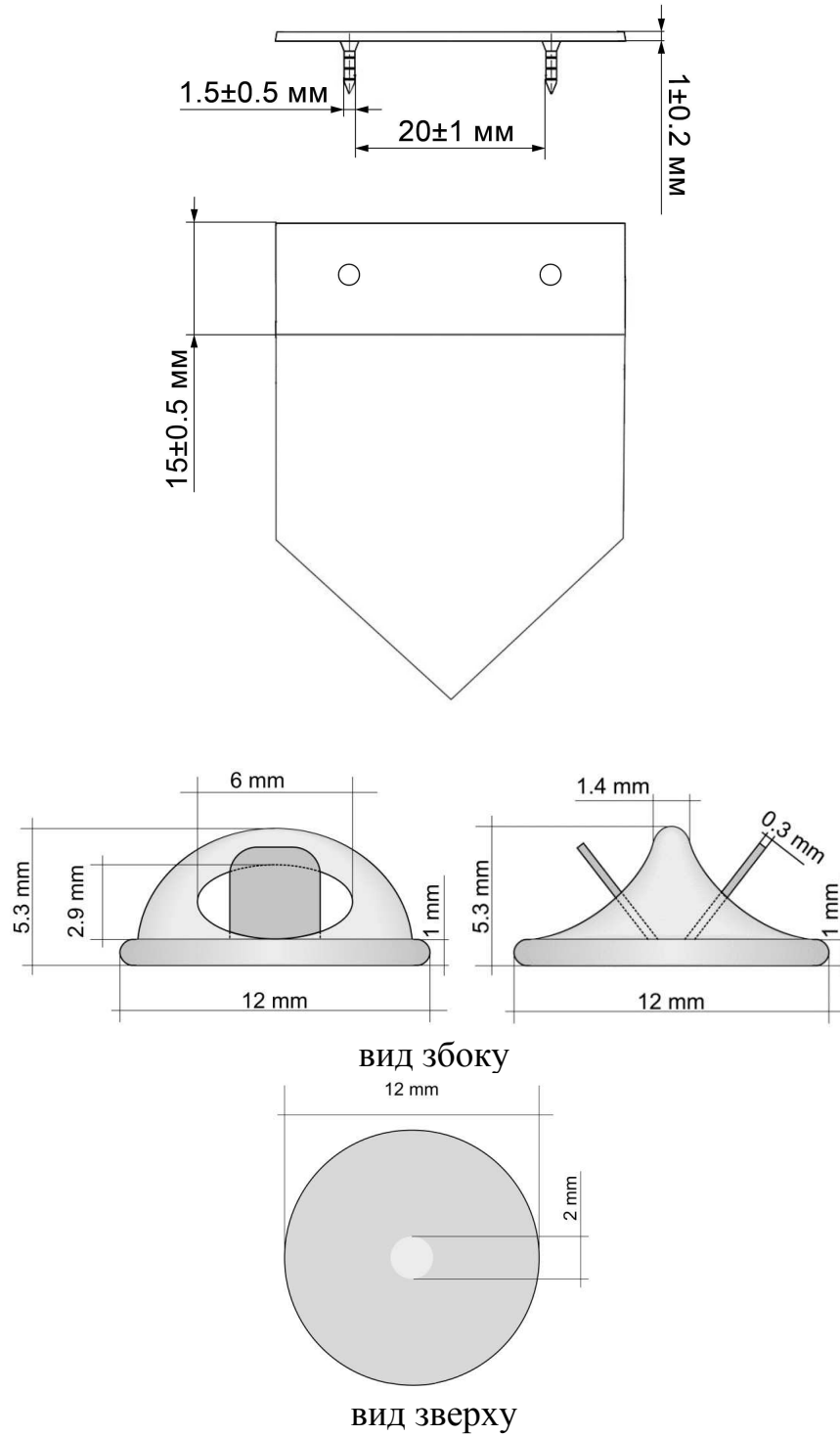
Рисунок Д2.1 – Зображення та розміри кріплення
