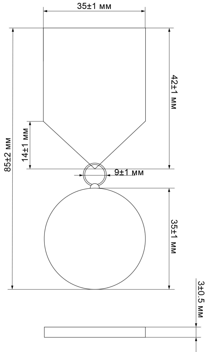
Рисунок Д1.1 – Розміри предмета
