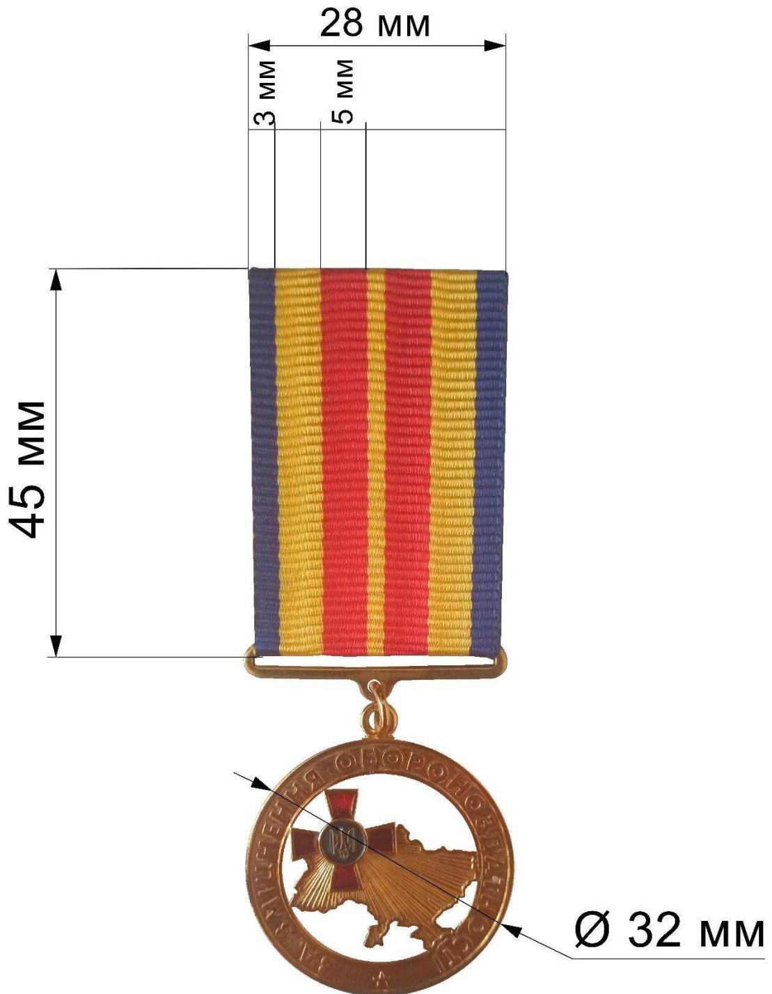
Рисунок 2 – Зовнішній вигляд та розміри медалей.
