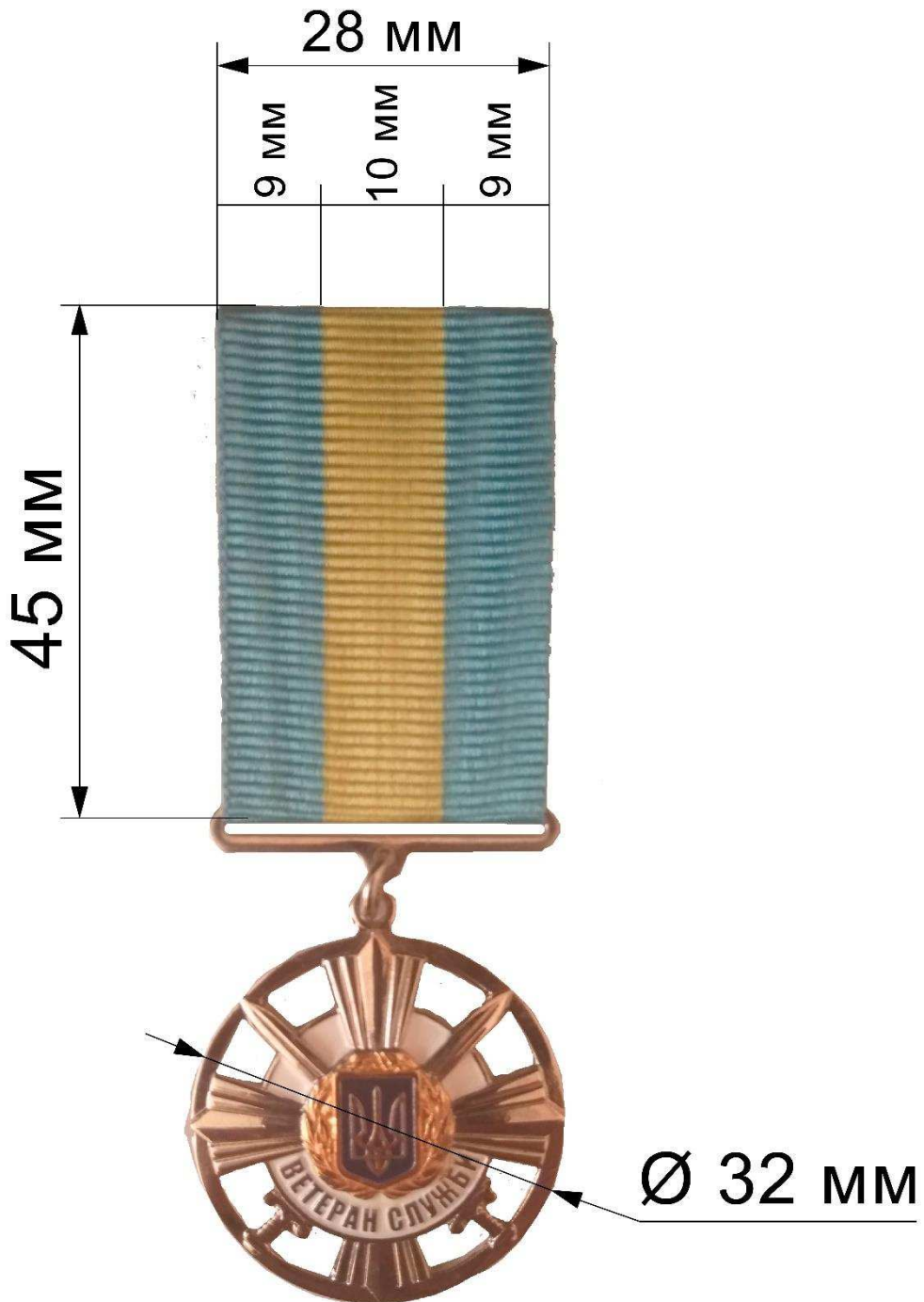
Рисунок 2 – Зовнішній вигляд та розміри медалей
