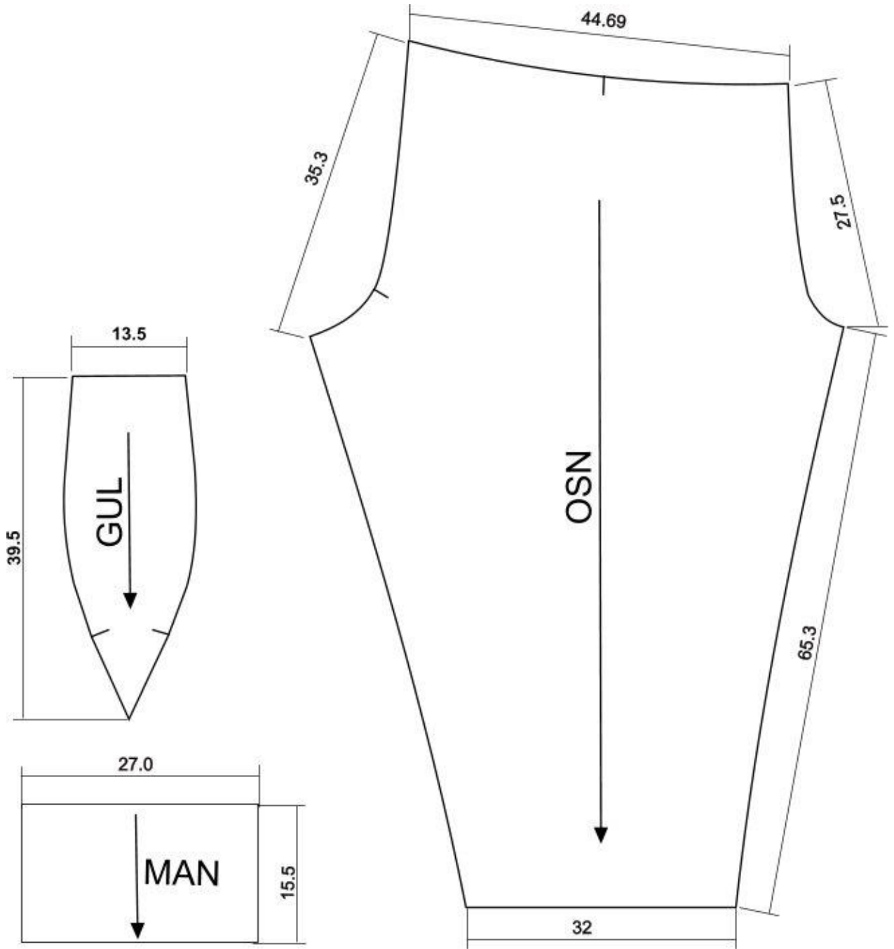
Рисунок Б8 — Ескізи лекал деталей виробу 2
