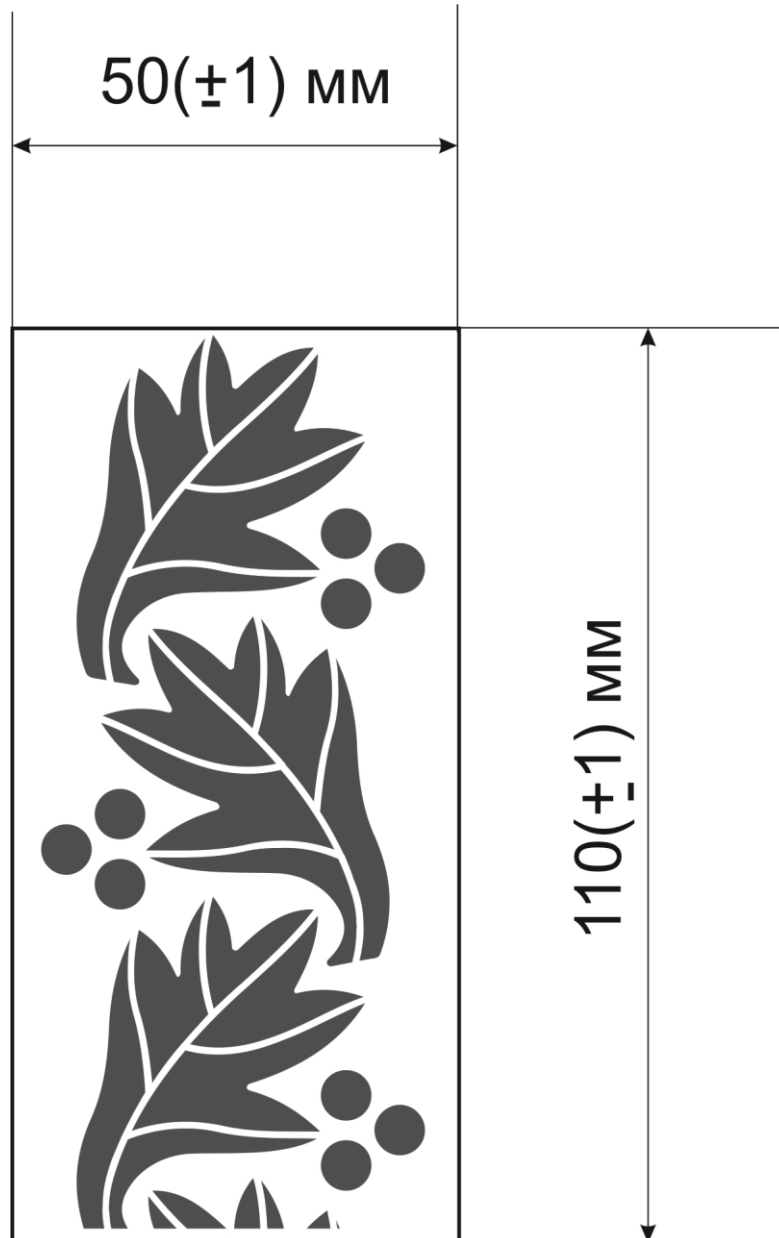
Рисунок Д1.1 – Розміри орнаменту
