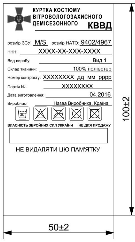
Рисунок 3 — Зовнішній вигляд етикетки виробу 1 та її розміри
