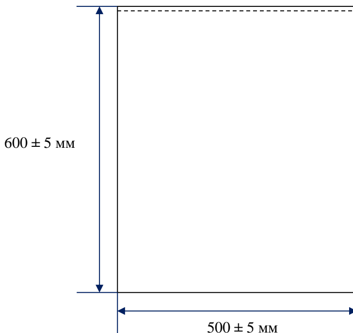
Рисунок 1. Загальний вигляд виробу
