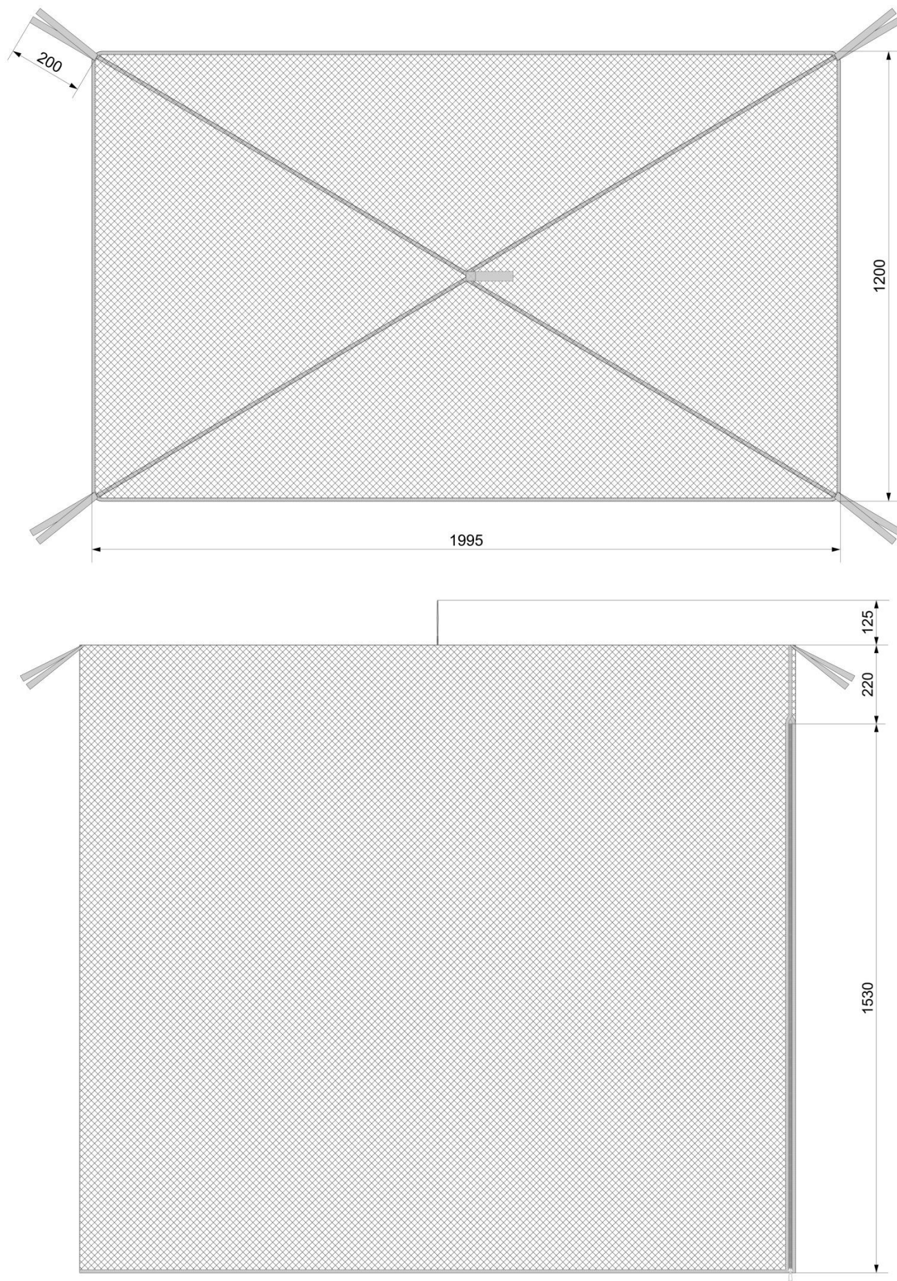
Рисунок 1. Загальний вигляд та лінійні виміри виробу
