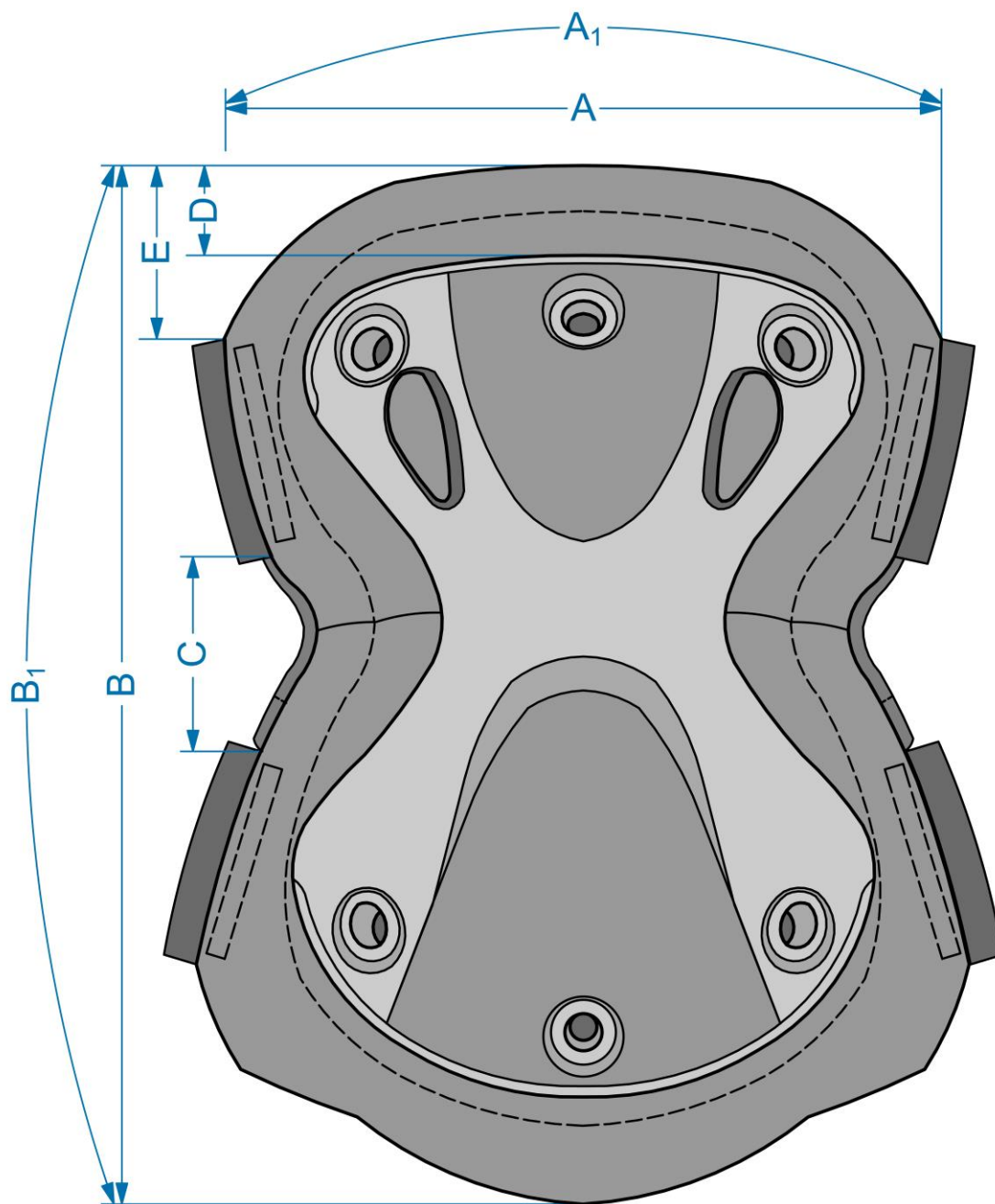
Рисунок Б.1— Лінійні виміри виробу
