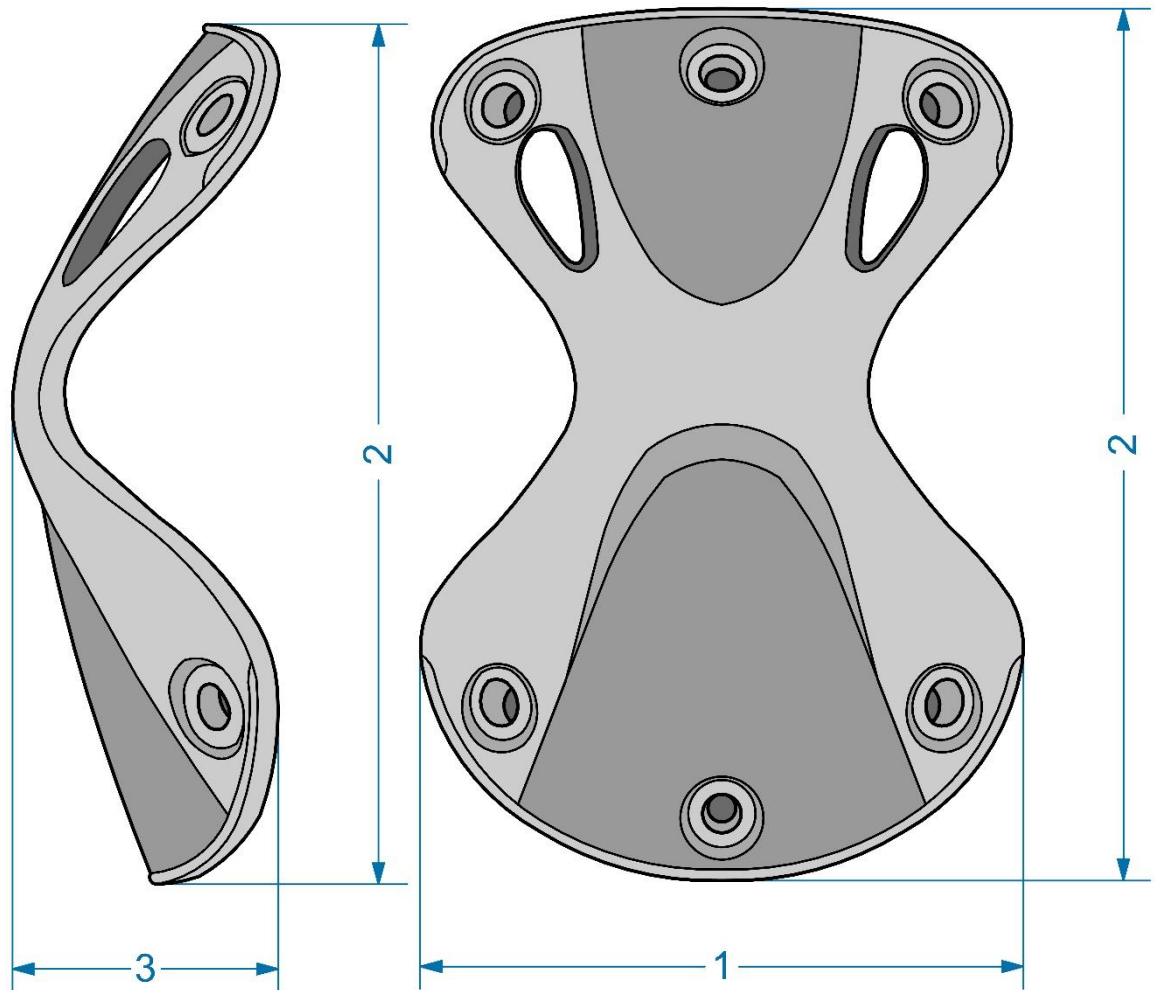
Рисунок Б.3 — Чашка з ударостійкого пластика
