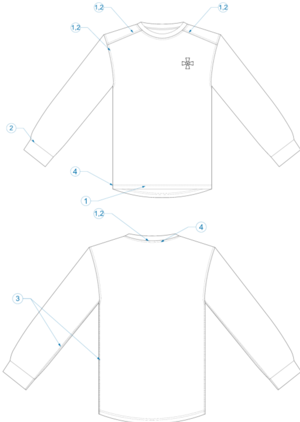
Рисунок Б5 — Позначення строчок виробу 1
