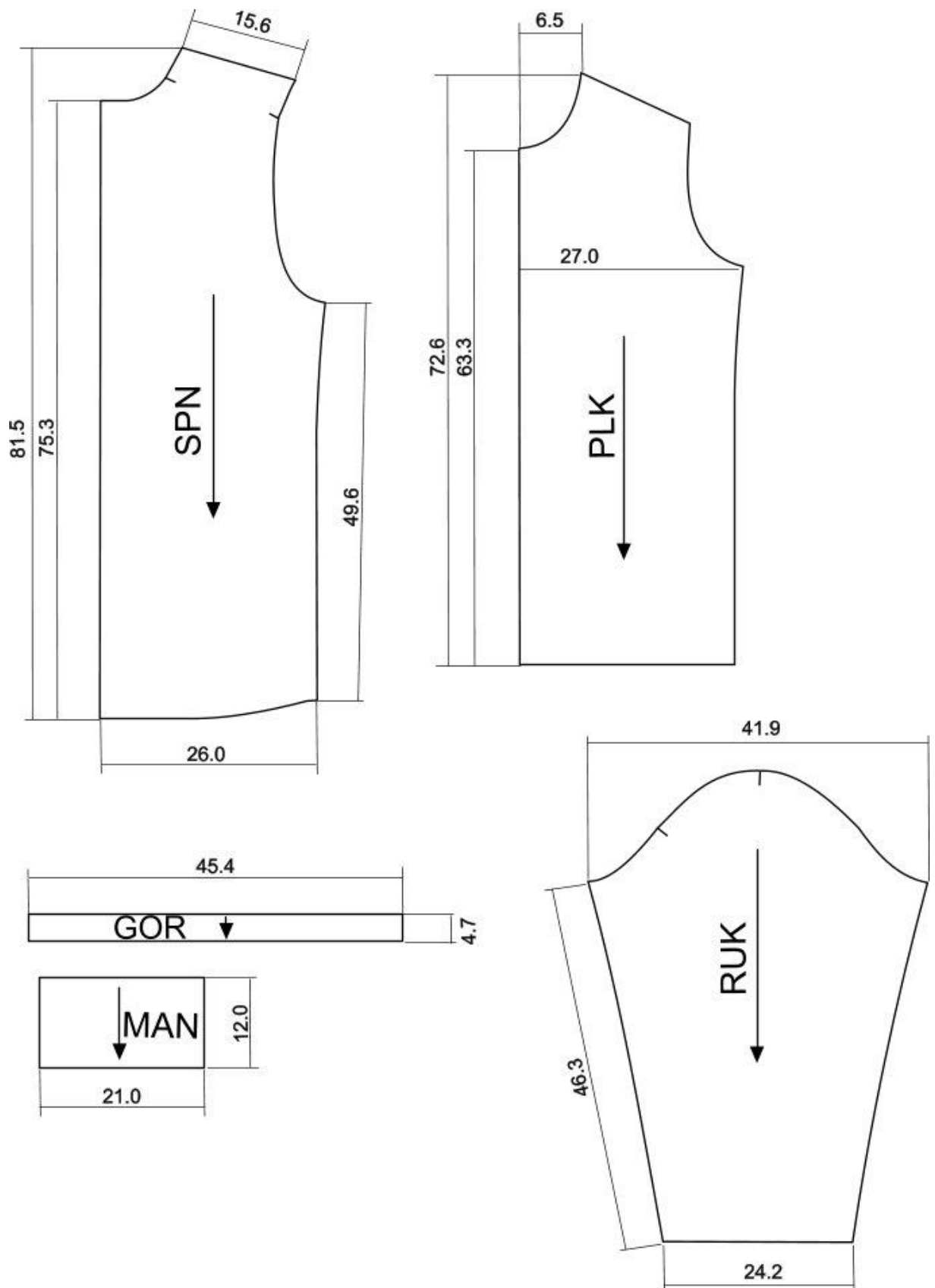
Рисунок Б7 — Ескізи лекал деталей виробу 1
