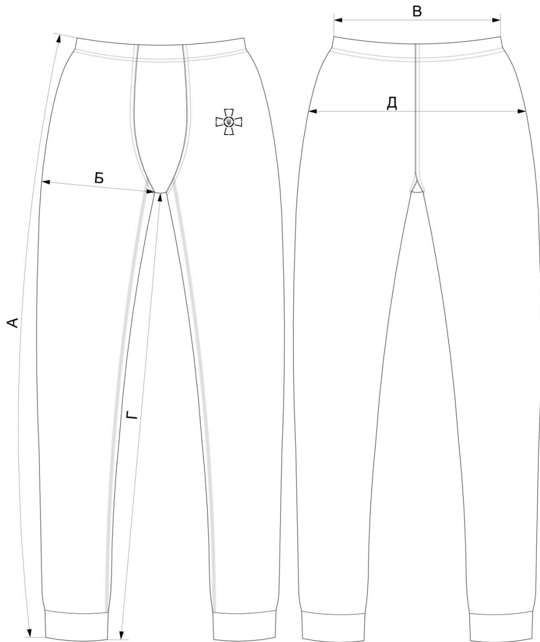
Рисунок Б2 – Лінійні виміри виробу 2
