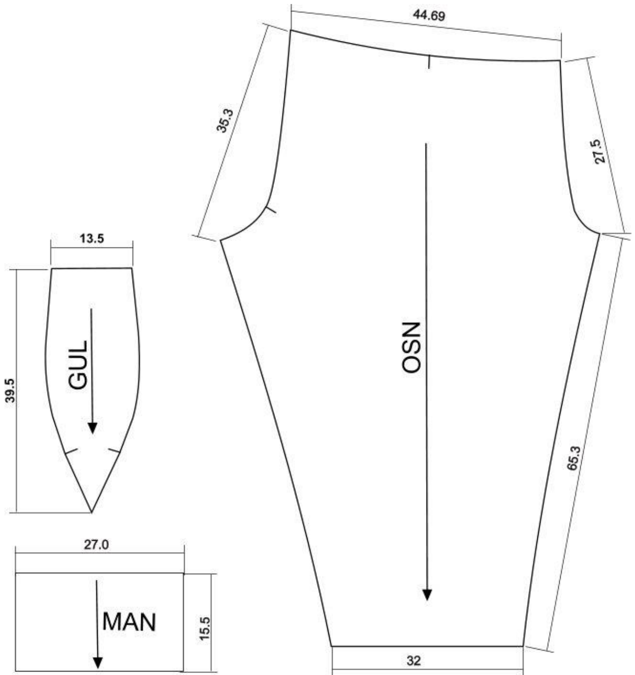
Рисунок Б8 — Ескізи лекал деталей виробу 2
